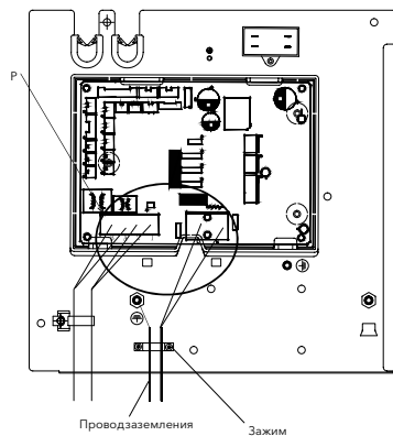
Увеличенный вид проводкиклеммной коробки(ТВ), деталь P
