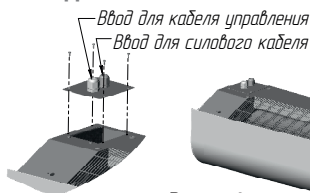
Рисунок 2. Воздушная завеса.
